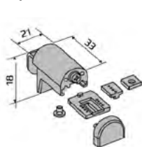
Кронштейн ПВХ
