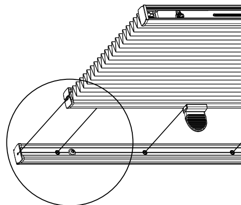
Регулировка натяжения троса в моделях P3xxx.
