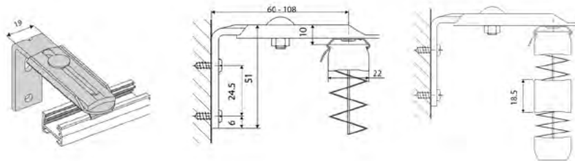
Кронштейн ПВХ
